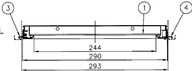
断面詳細図 (1/3)
