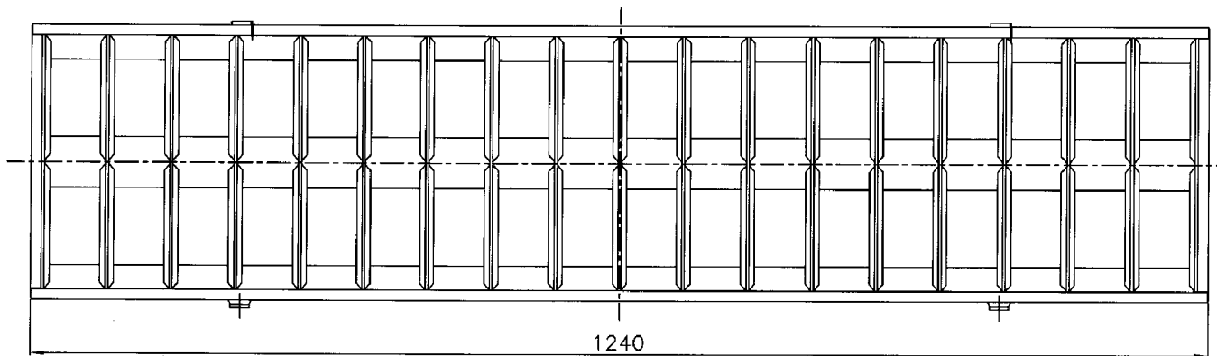
断面詳細図 (1/2)
