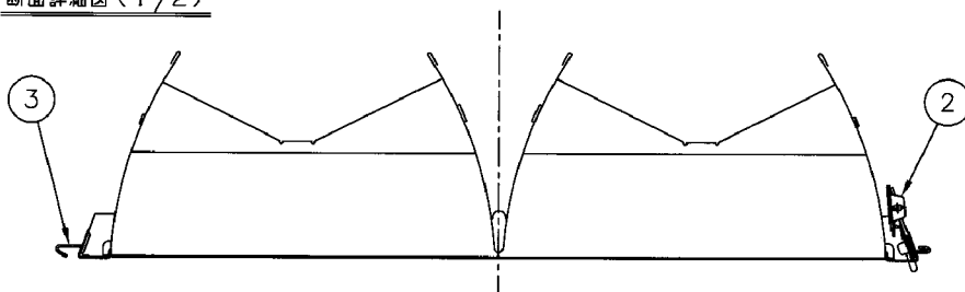
断面詳細図 (1/2)
