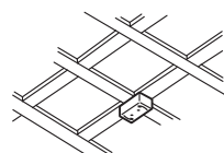
格子天井
