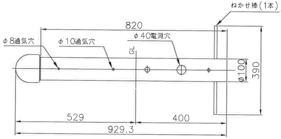
外観図
