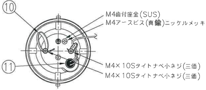
A-A断面図
