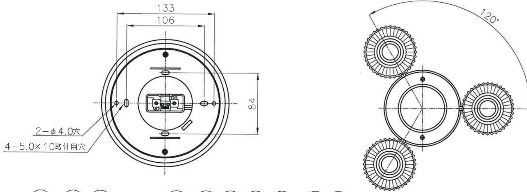
下面図：1/5
