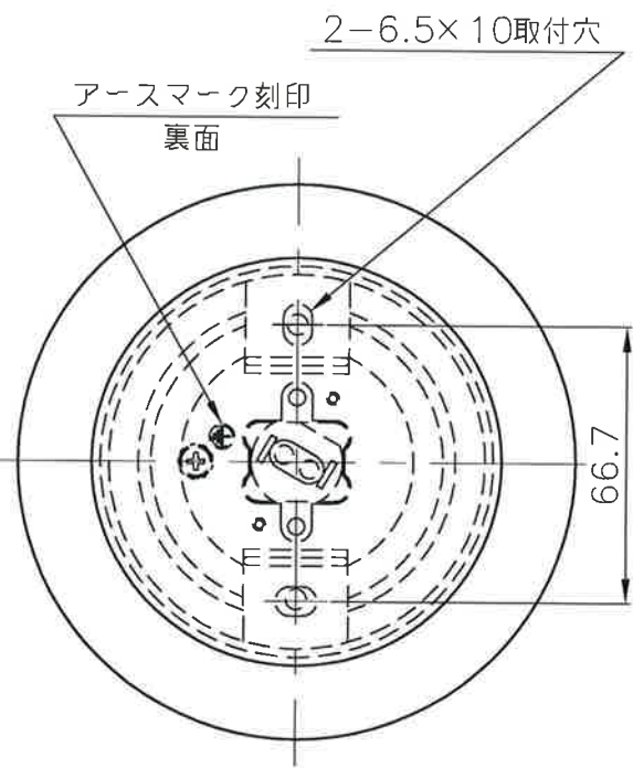
< 本体 (取付部) >
