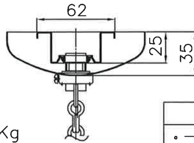
断面詳細図1/3
