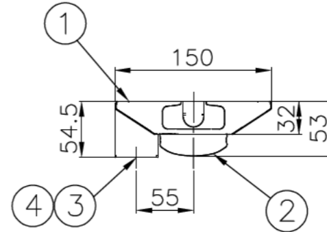
側面詳細図
