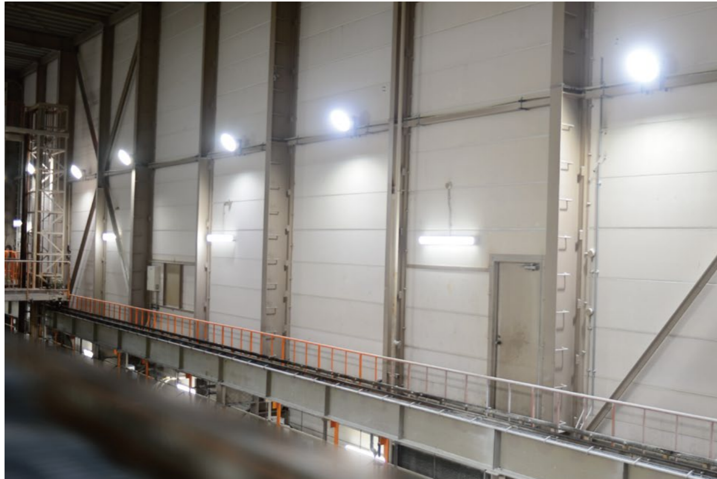
高天井用LED照明器具 高温環境対応形（耐腐食仕様） DRGE15H05(HTS)G/N-ZJX8 平均消費電力：99W
