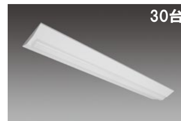
30台 LED一体型ベース照明 Nuシリーズ 逆富士形230mm幅 MVB4103/52N4-N8 定格消費電力: 31.5W
