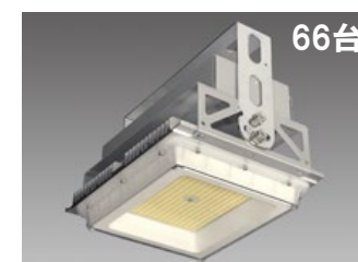
66台 高天井用LED照明器具 DRGE17H41S/N-P8 定格消費電力: 86W
