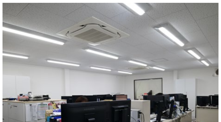
高天井用LED照明器具 電源別置型 DRCE17H32K/N-ZJX8 定格消費電力:100W
