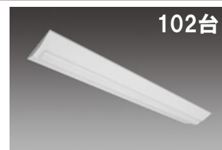
102台 LED一体型ベース照明器具 40形 Nuシリーズ 逆富士形230mm幅 MVB4103/40W4-N8 定格消費電力:24.7W
