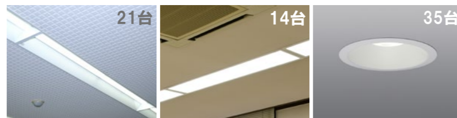
LED一体型ベース照明 110形 埋込下面開放形 (特注品) 定格消費電力:83.6W
