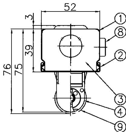
断面图
