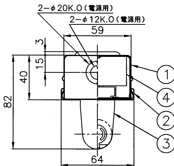
断面詳細図
