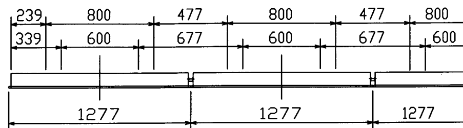
埋込連結使用例
