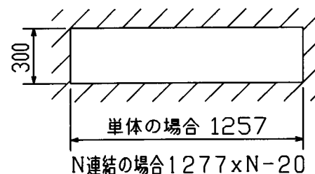
埋込穴寸法
