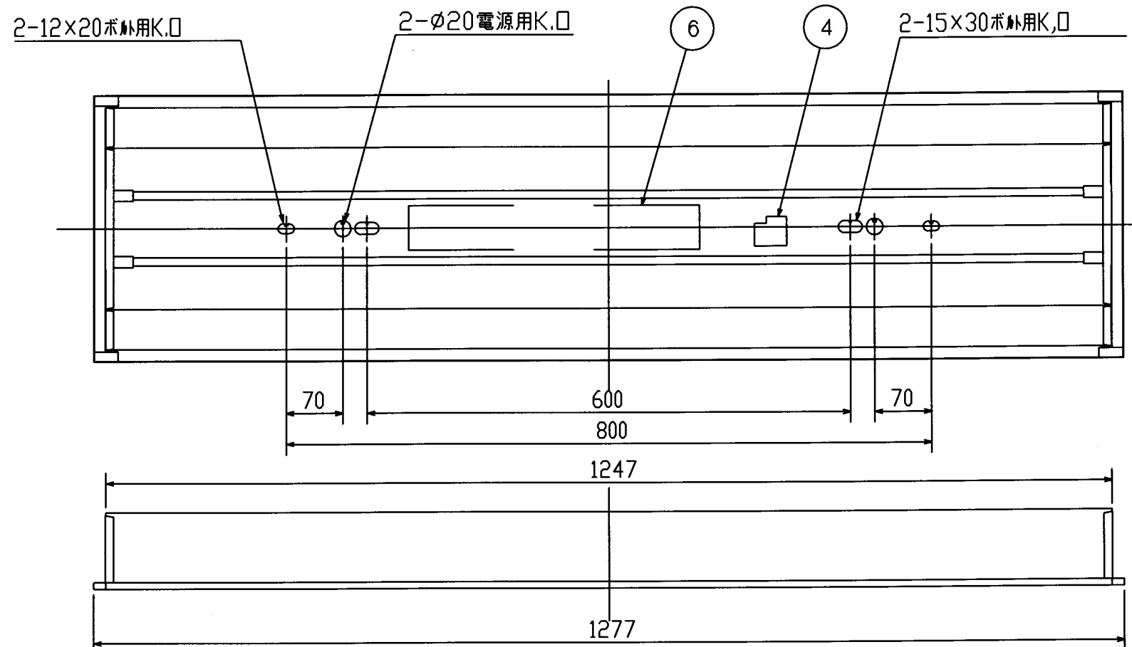
埋込連結使用例
