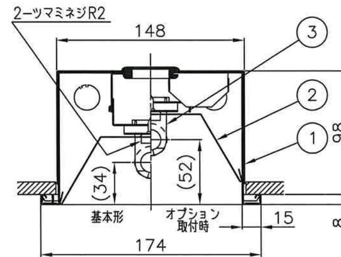
断面詳細図 (1/3)
