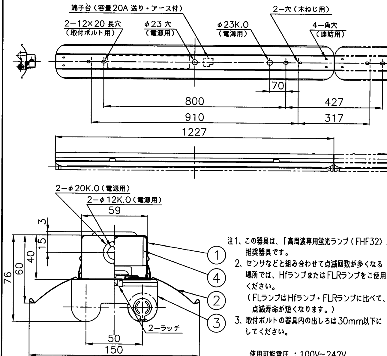
断面詳細図
