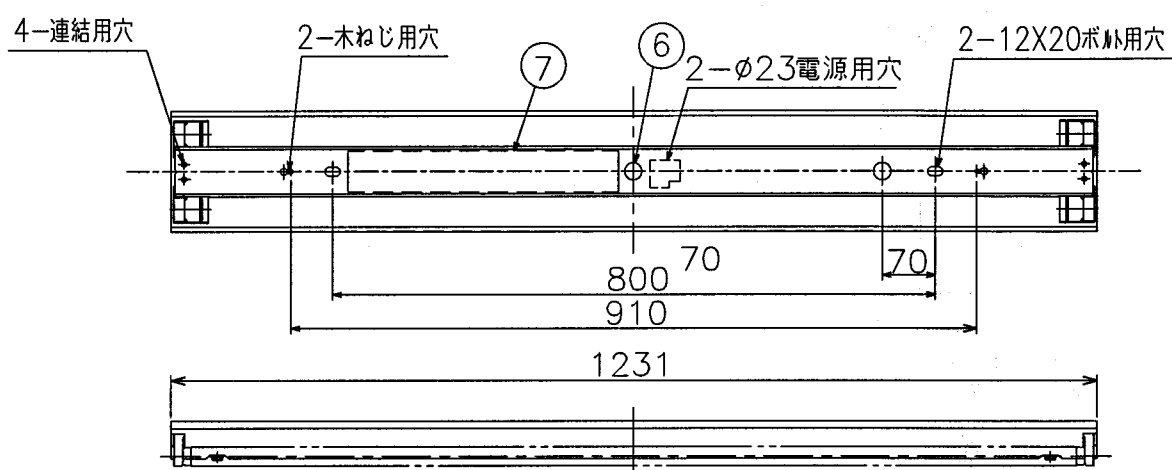
直付連結使用例
