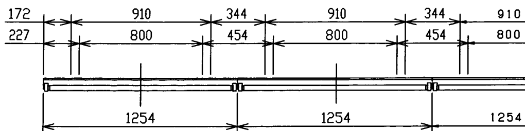
直付連結使用例
