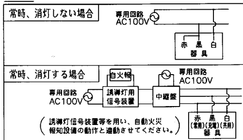
結線図
