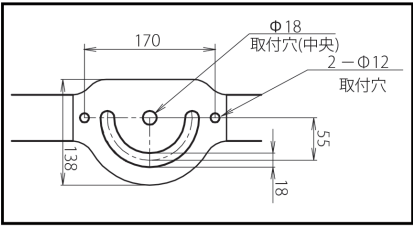
取付穴詳細
