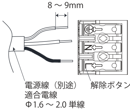
電源端子台
