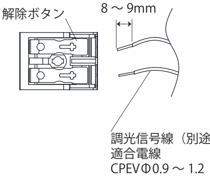
調光端子台
