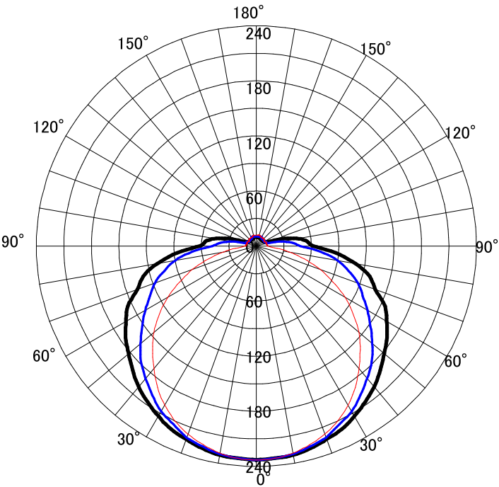
配光曲線図 光度 cd/1000lm — A-A — B-B — C-C
