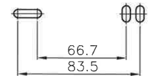
取付寸法 (mm)
