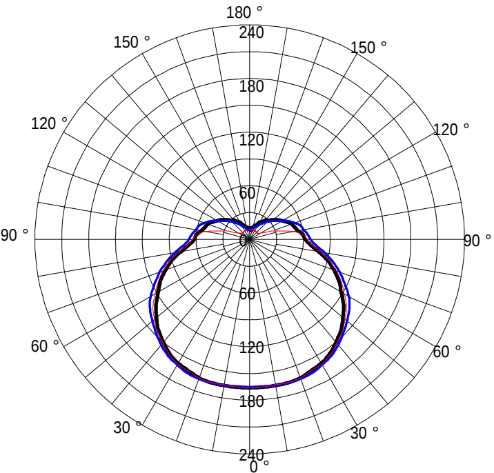
配光曲線図 光度 cd/1000lm A - A B - B C - C
