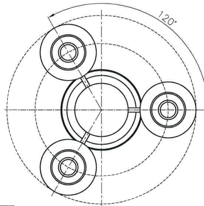
下面図：1/5
