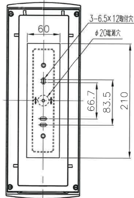
<本体（取付部）>
