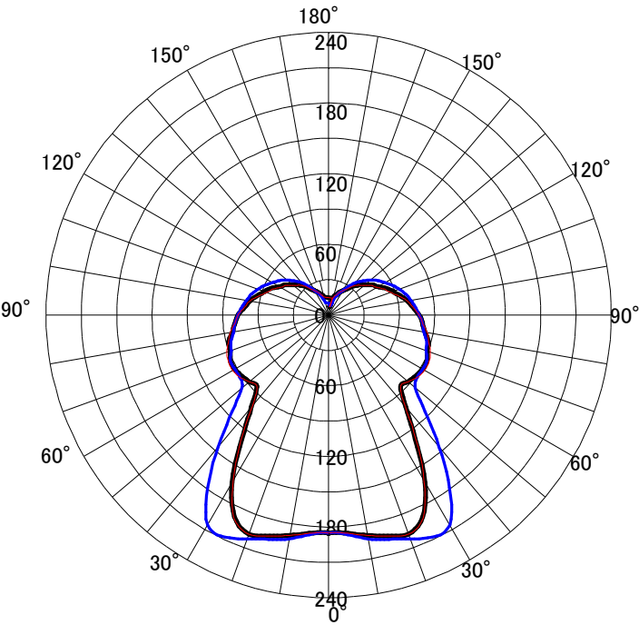
配光曲線図 光度 cd/1000lm
