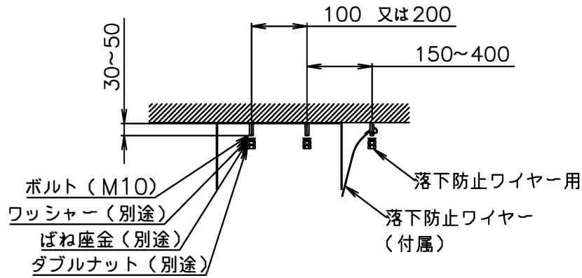
取付設置図
