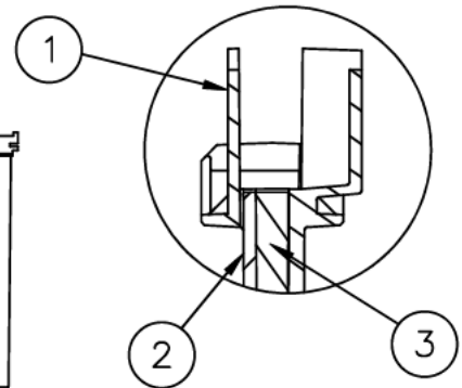
A部断面拡大図
