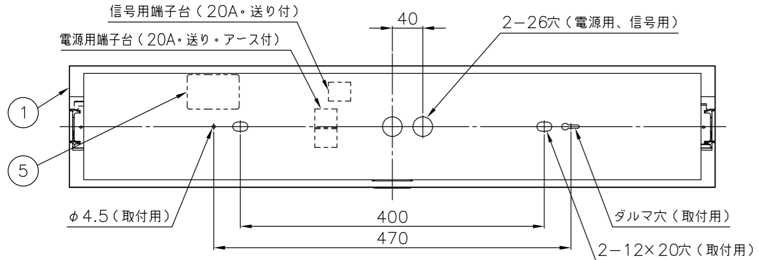
背面図
