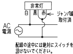
配線図
