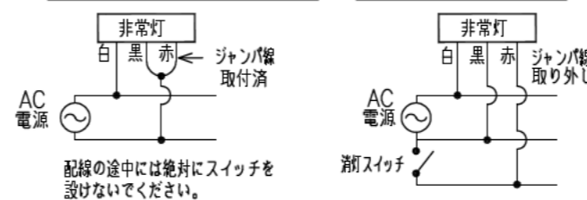
配線図
