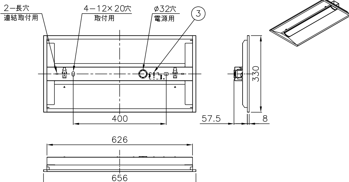
埋込み穴寸法 300×639 (単体)
