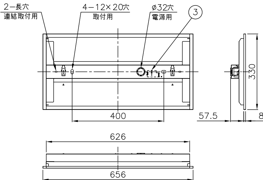
埋込み穴寸法 300×639 (単体)
