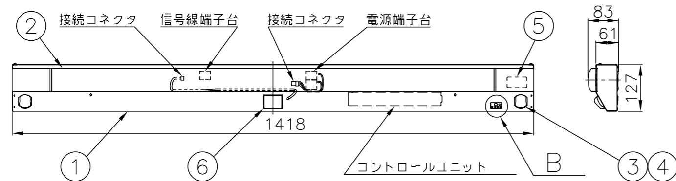
配線図
