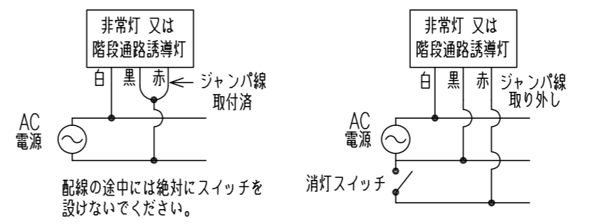
配線図 A 単相2線式(2線引) (常時にライトユニットを消灯しない場合の例) B 単相2線式(3線引) (常時にスイッチ消灯する場合の例)
