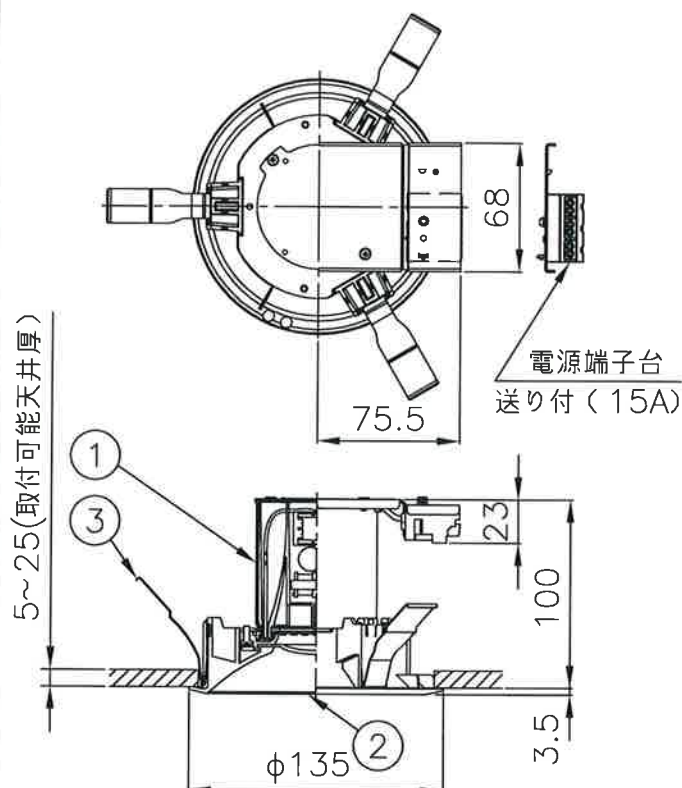
組合形名 MRB10028W2/L-8 ライトユニット DRU10028/L-8 (0643-4066) 反射板枠 MRB-W2ワ (0643-3763)
