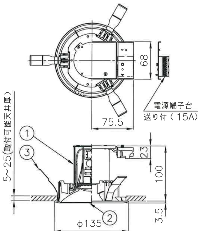
組合形名 MRB06028W2/N-8 ライトユニット DRU06028/N-8 (0643-4067) 反射板枠 MRB-W2ワク (0643-3763)
