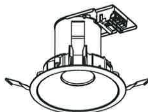
組合形名 MRB06028W2/N-8 ライトユニット DRU06028/N-8 (0643-4067) 反射板枠 MRB-W2ワク (0643-3763)
