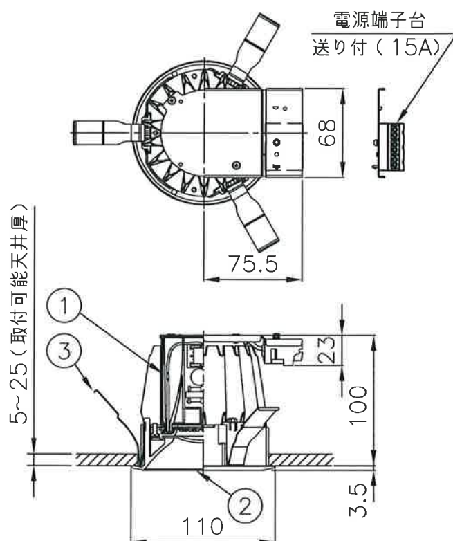
組合形名 MRB20028W1/WW-8 ライトユニット DRU20028/WW-8 (0643-4070) 反射板枠 MRB-W1ワク (0643-3764)
