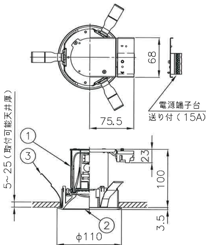
組合形名 MRB06028W1/WW-8 ライトユニット DRU06028/WW-8 (0643-4076) 反射板枠 MRB-W1ワク (0643-3764)
