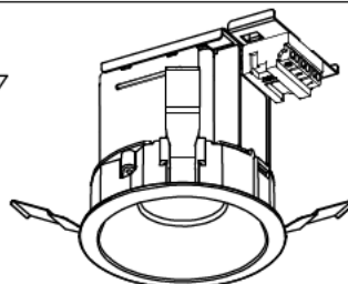
組合形名 MRB20029W1/N-8 ライトユニット DRU20029/N-8 (0643-4562) 反射板枠 MRB-W1ワ (0643-3764)
