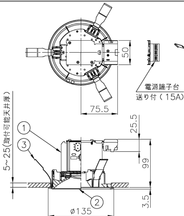
組合形名 MRB10029W2/N-8 ライトユニット DRU10029/N-8 (0643-4570) 反射板枠 MRB-W2ワ (0643-3763)
