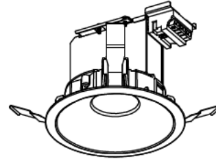
組合形名 MRB06029W2/L-8 ライトユニット DRU06029/L-8 (0643-4577) 反射板枠 MRB-W2ワク (0643-3763)
